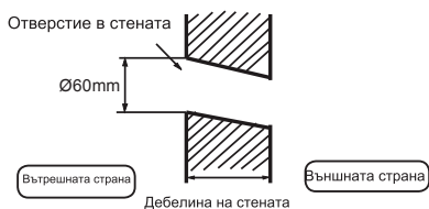
(Разрез на отворието в стената) ⓐ Отворието за тръбопровод
